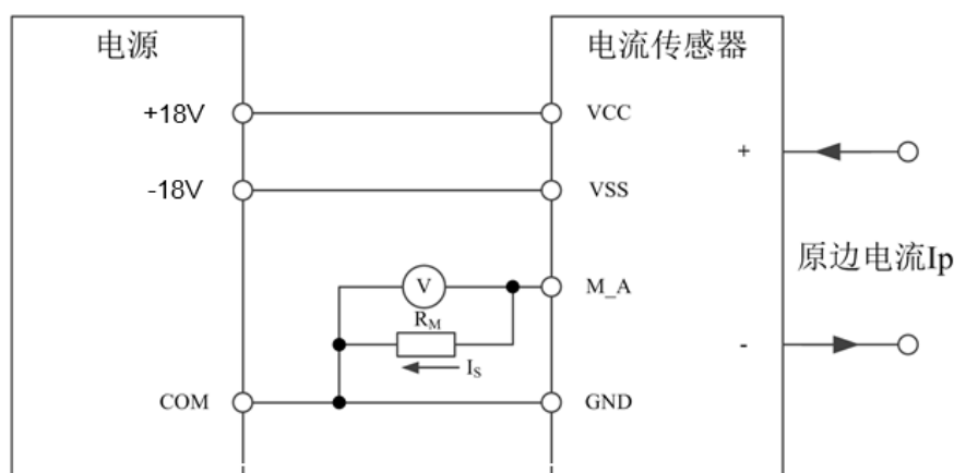
图 3: 电气连接图
