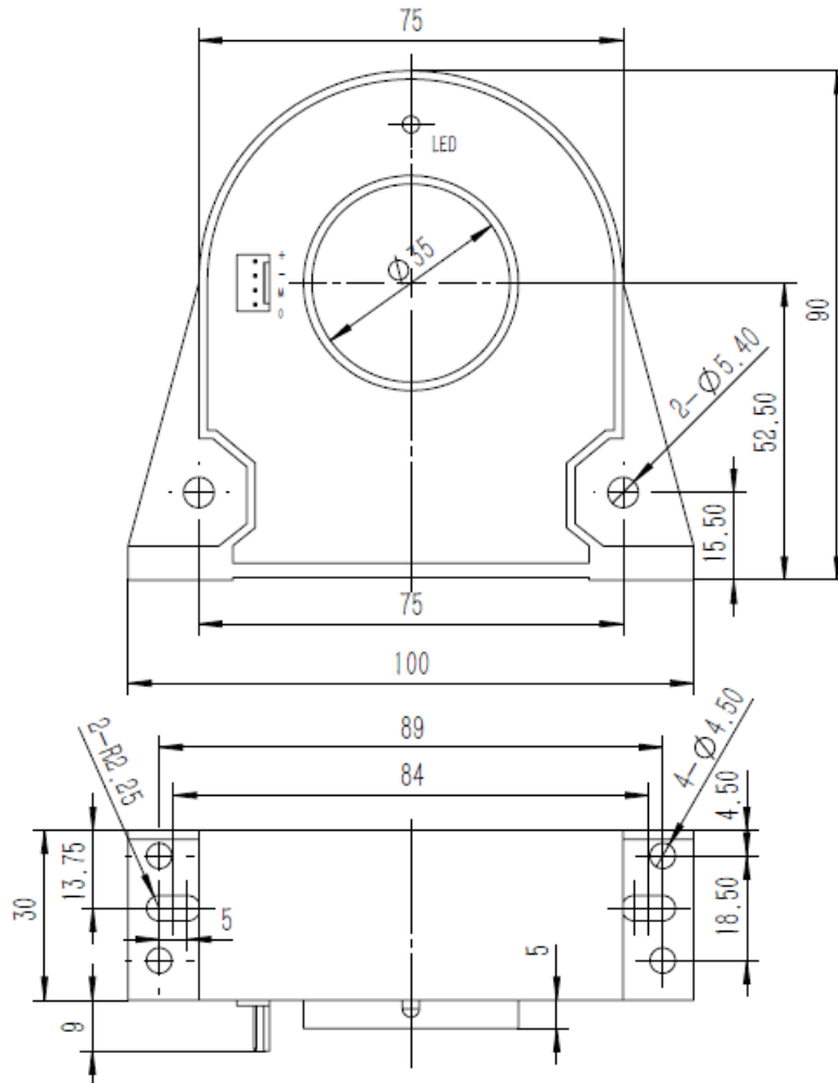
图 1 外形图
