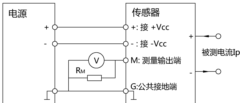
电气连接图
